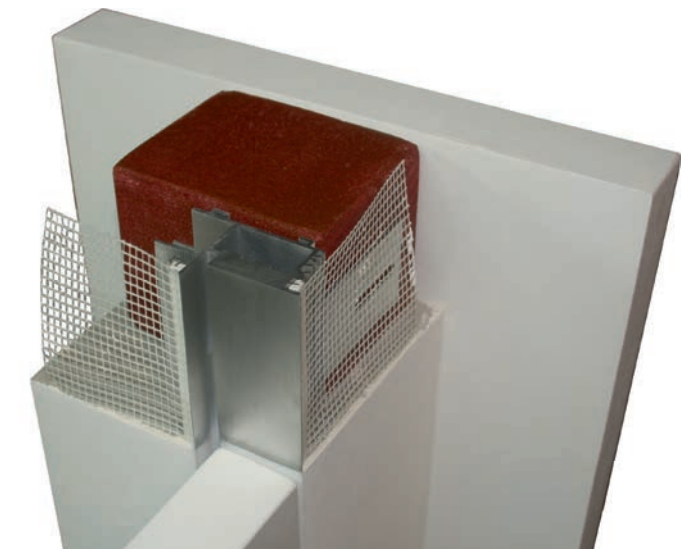
Detailansicht TCT
